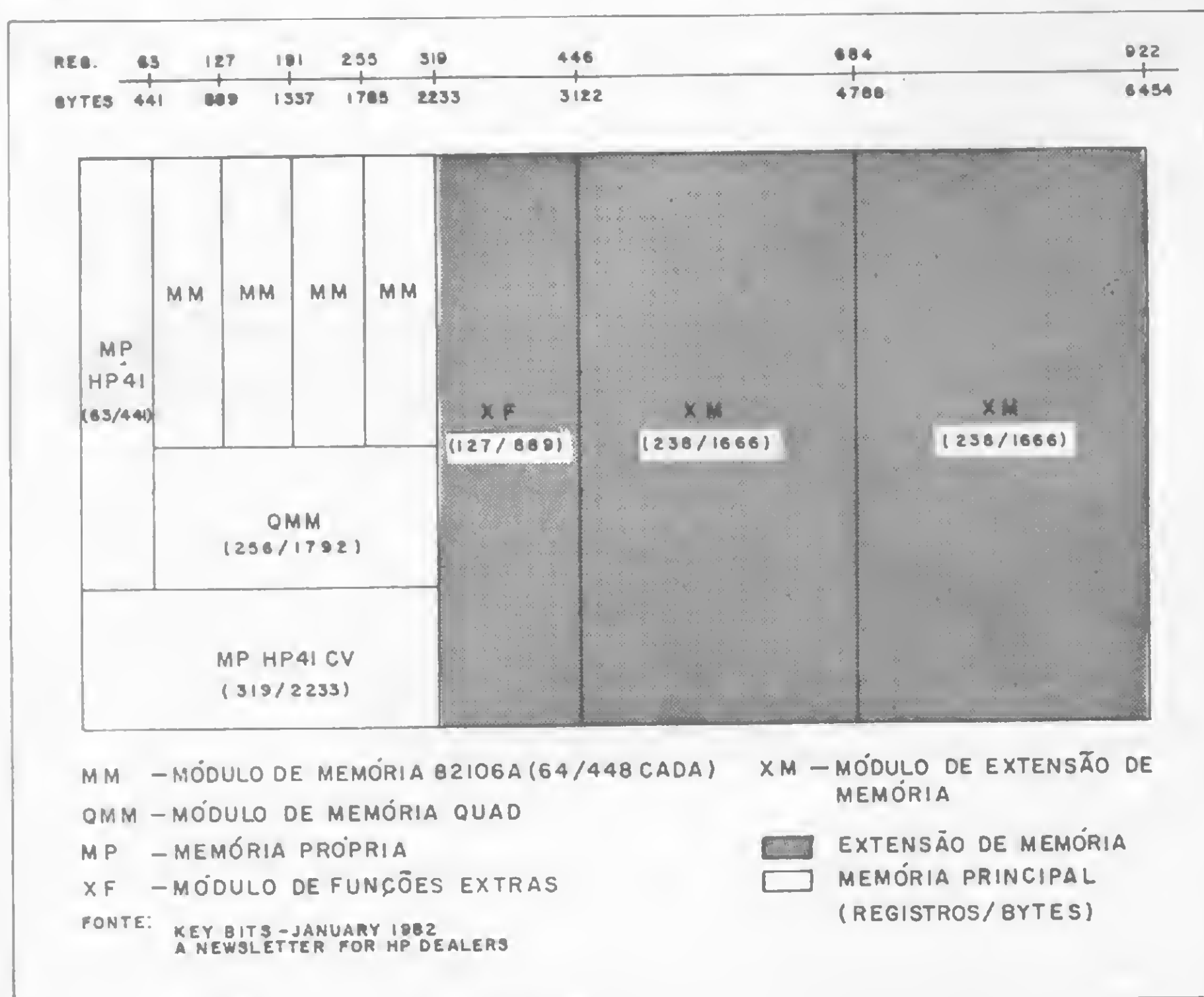
Figura 1 - Esquema da partição de memória.
